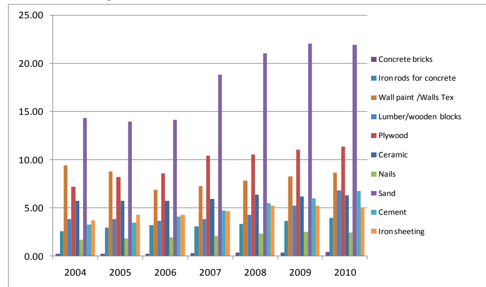
Grafiku 14: Komponenti Kustu Harii Uma
